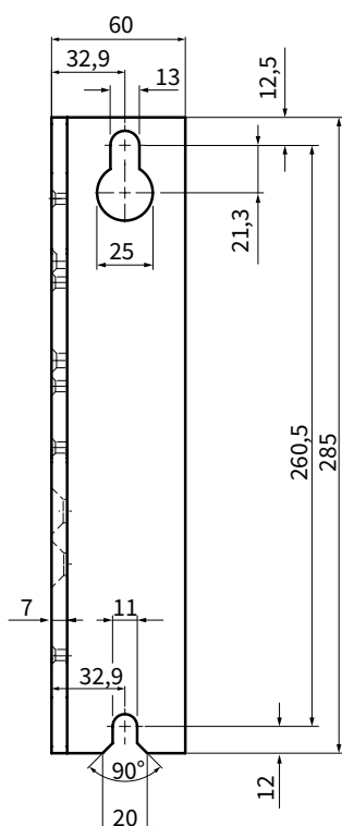
vooraanzicht muursteun links
