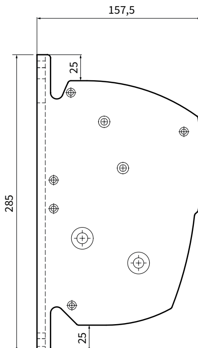
zij aanzicht muursteun links
